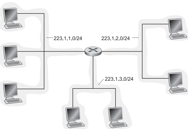
Figura 4.16 • Direcciones de subred.
