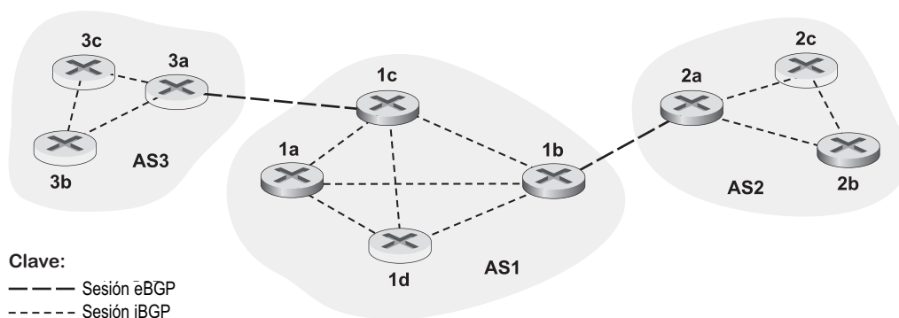
Figura 4.40 • Sesiones eBGP e iBGP.
