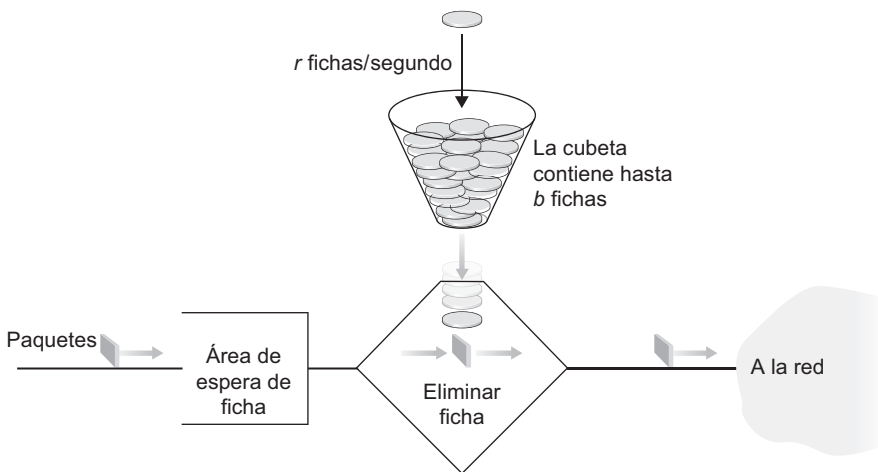
Figura 7.27 • El controlador de la cubeta con pérdidas.
