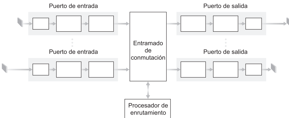
Figura 4.6 • Arquitectura de un router.
