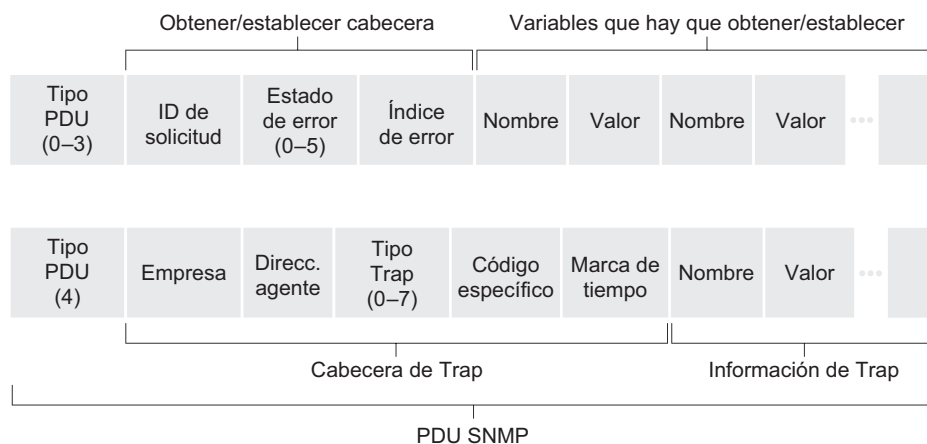
Figura 9.4 • Formato de la PDU de SNMP.
