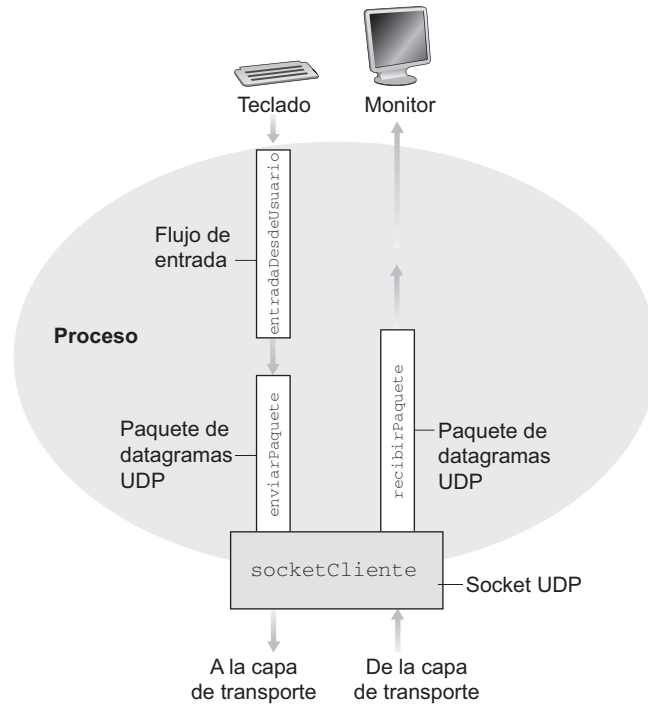
Figura 2.33 • UDPCliente tiene un flujo; el socket acepta paquetes del proceso y suministra paquetes al proceso.
