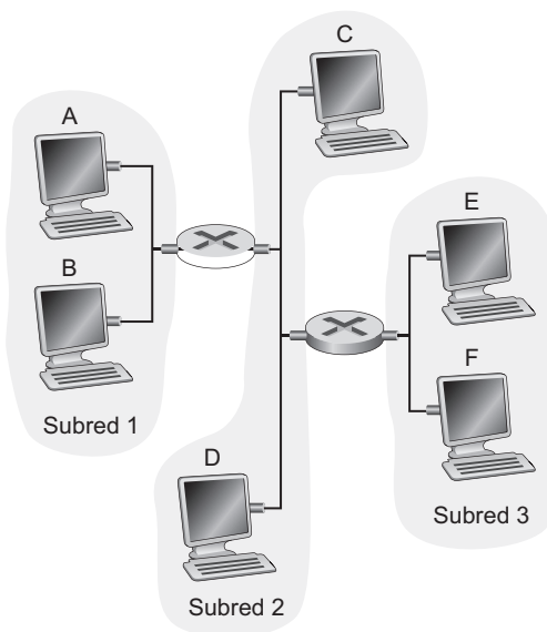
Figura 5.38 • Tres subredes interconectadas mediante routers.
