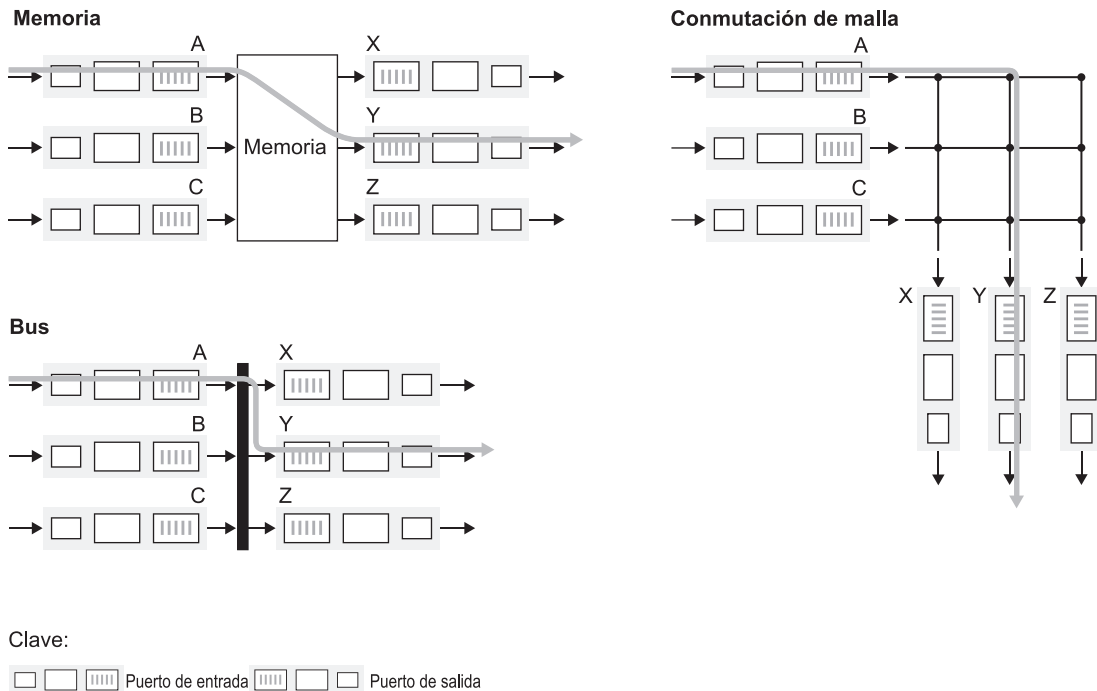
Figura 4.8 • Tres técnicas de conmutación.
