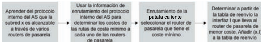
Figura 4.33 • Pasos para añadir a la tabla de reenvío de un router un destino externo al sistema autónomo.
