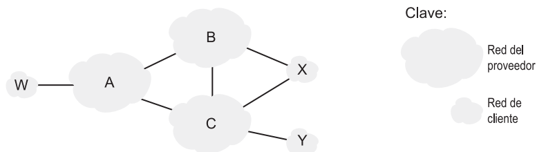
Figura 4.42 • Un escenario BGP simple.
