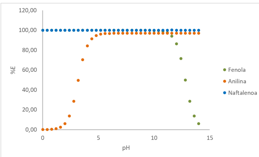
1. Irudia. Erauzketa likido-likidoa; Fenola, anilina eta naftalenoaren banaketa disolbatzaile desberdinak erabiliz.
