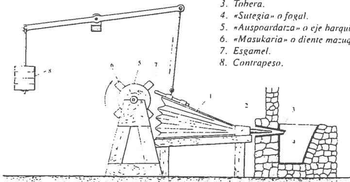
ALIMENTADOR DE AIRE CON FUELLES
